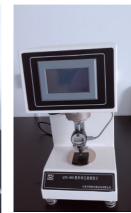
QYS-96B 塑料球压痕硬度计
