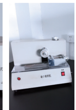
缺口制样机
