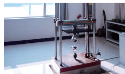
万能试验机 10吨
